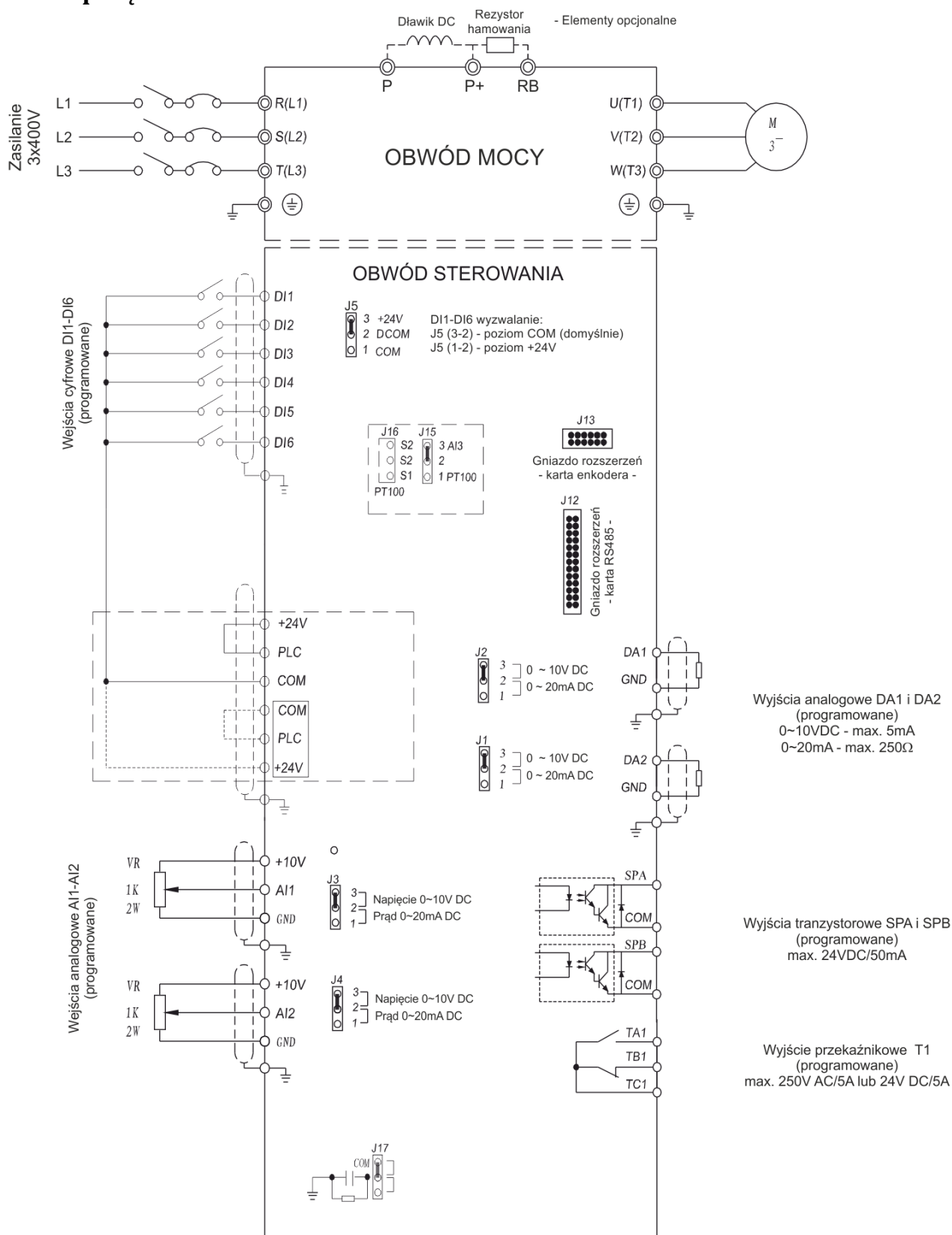
Rys. 4) Schemat podłączenia falownika FA-3HX007 ... FA-3HX075
