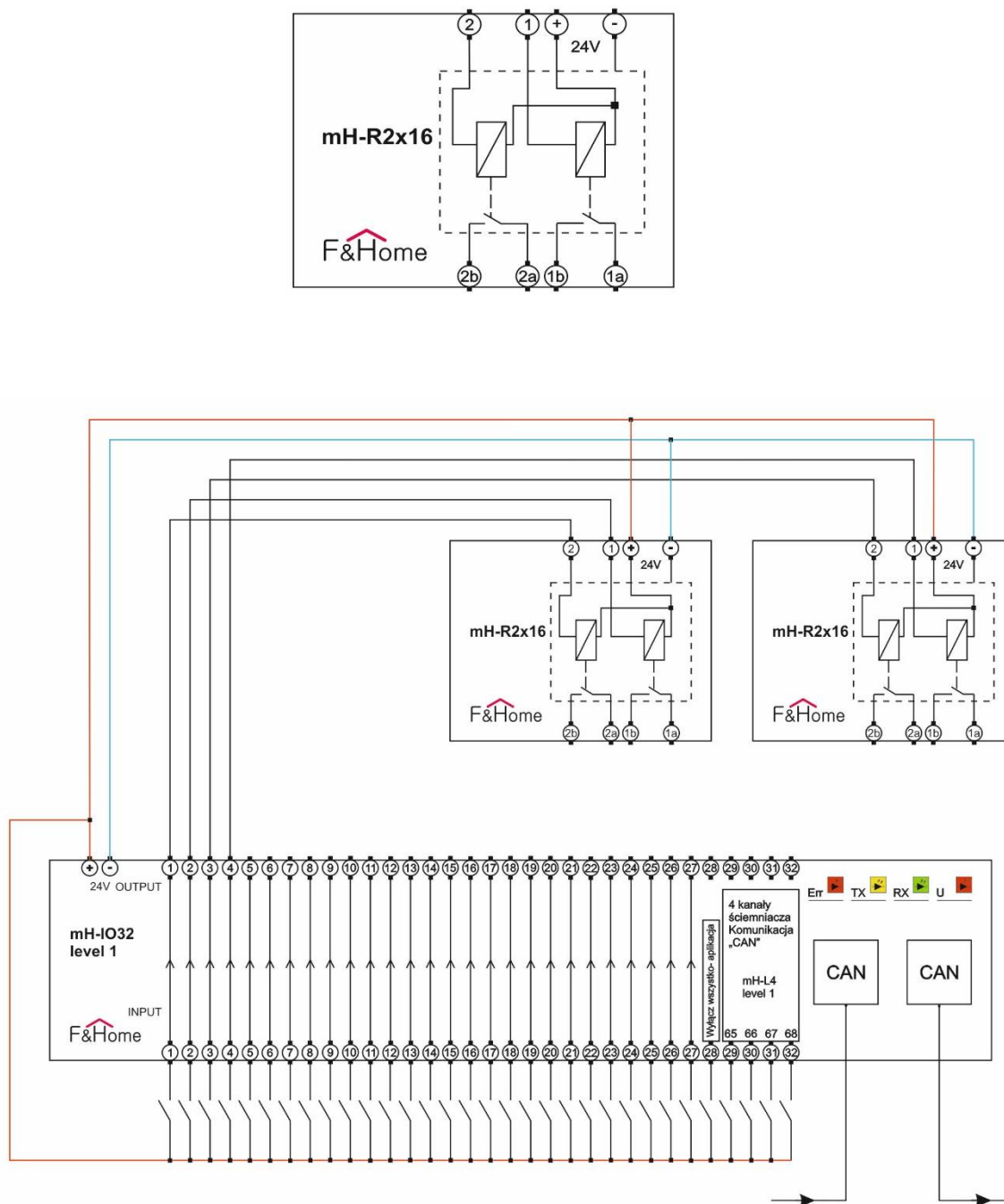
Podłączenie modułu wykonawczego (przełączników – mH-R2x16) do modułu wejść-wyjść.
