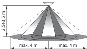
Wysokość instalacji czujnika i regulowany zasięg pola detekcji czujnika
