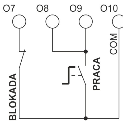
b) Sterowanie dwuprzewodowe
