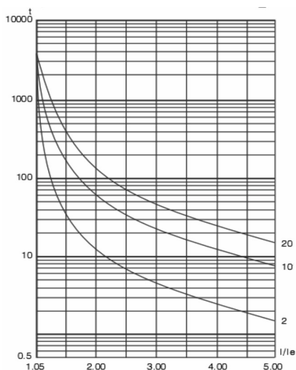
Rys. 24: Charakterystyki zabezpieczenia termicznego
