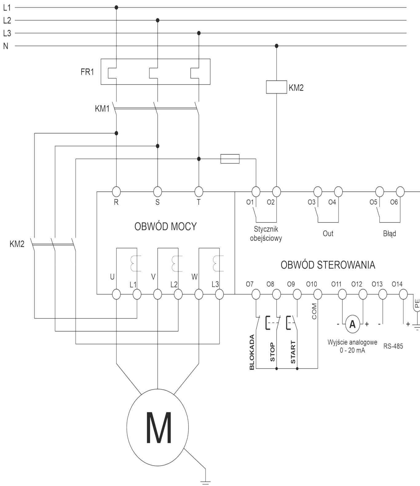
Rys. 4: Schemat połączeń
