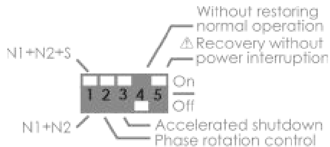
Rys. 8) Przełączniki konfiguracyjne
